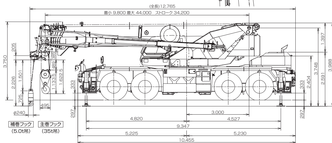
主巻フック
